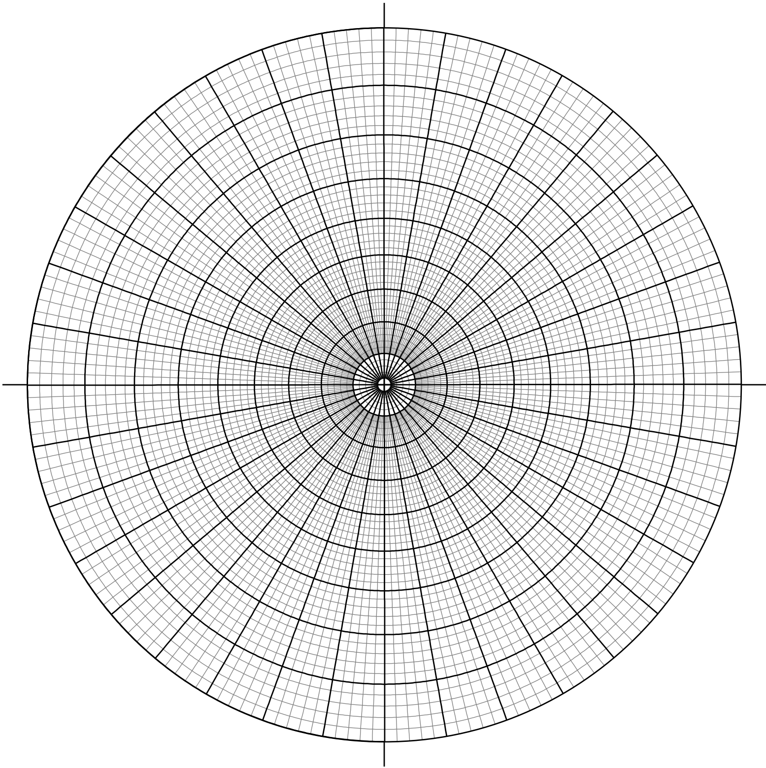
Polständiges Netz Stereographische Projektion (winkeltreu, Wulff'sches Netz)
