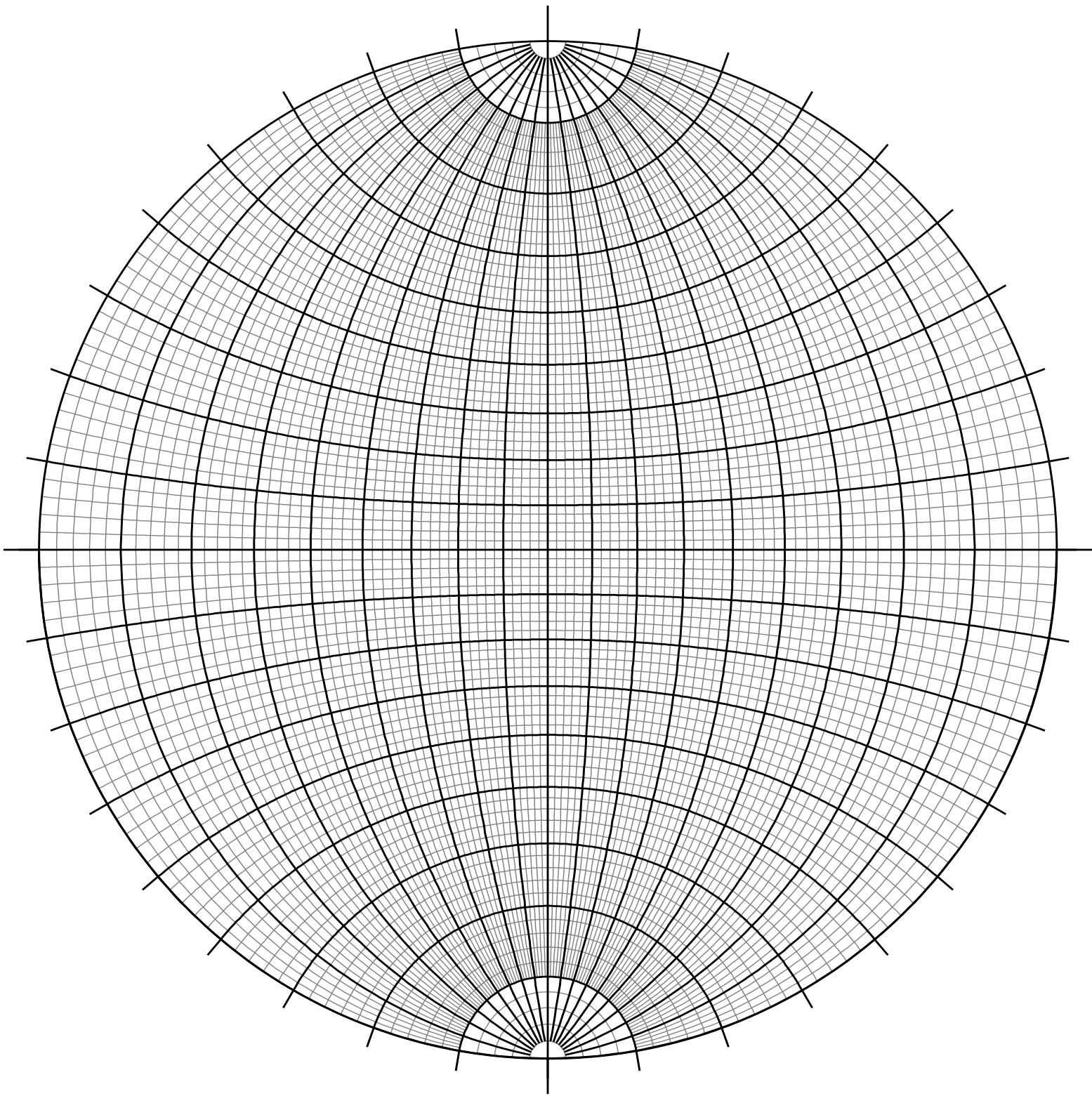
Stereographische Projektion (winkeltreu, Wulff'sches Netz)
